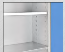
Fachböden verstellbar in 25 mm Schritten
